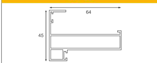
DOOR FRAM ( INSIDE OPENING )
