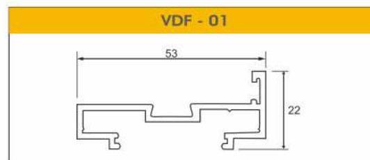
SLIM DOOR FRAME
