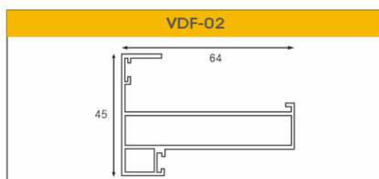
DOOR FRAM ( INSIDE OPENING )
