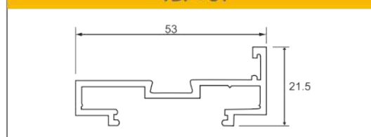
SLIM DOOR FRAME
